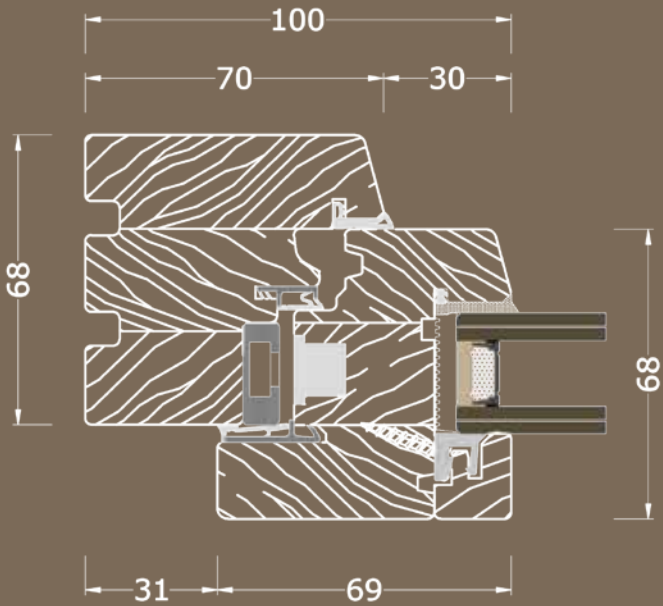
NODO LATERALE
