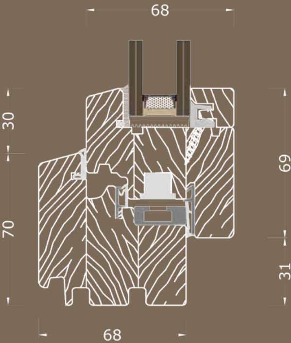
NODO INFERIORE
