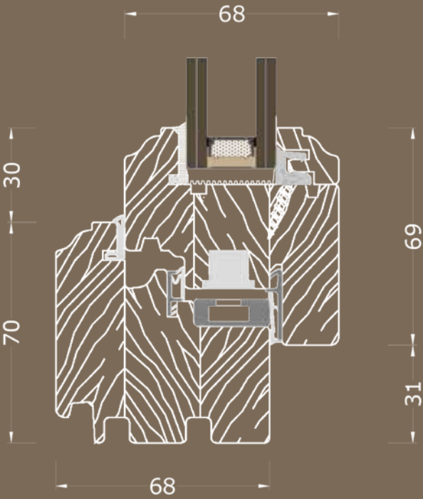
NODO INFERIORE
