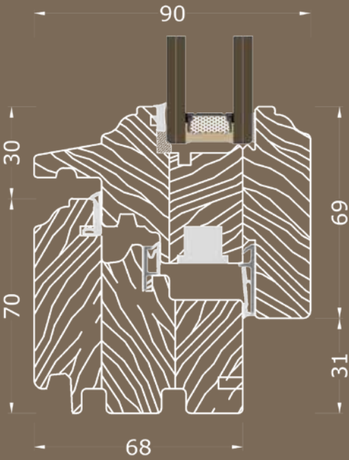
NODO INFERIORE
