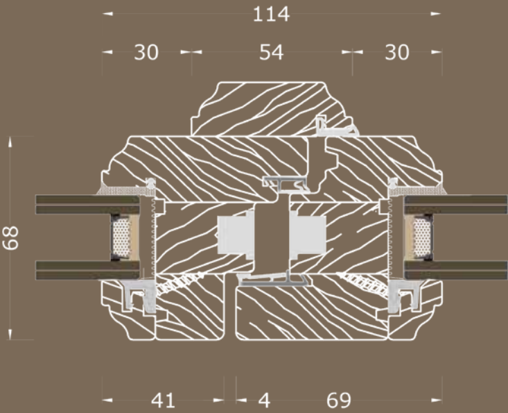
NODO CENTRALE
