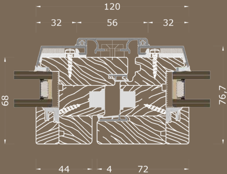
NODO CENTRALE
