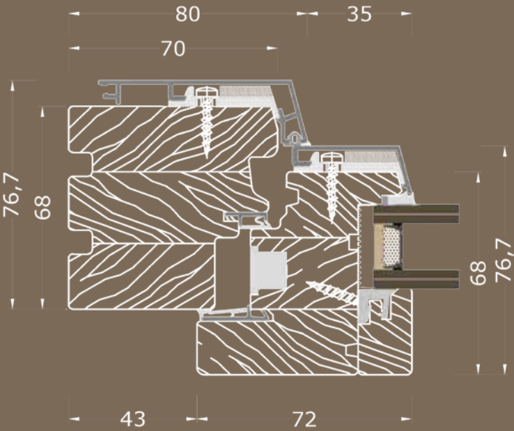
NODO LATERALE
