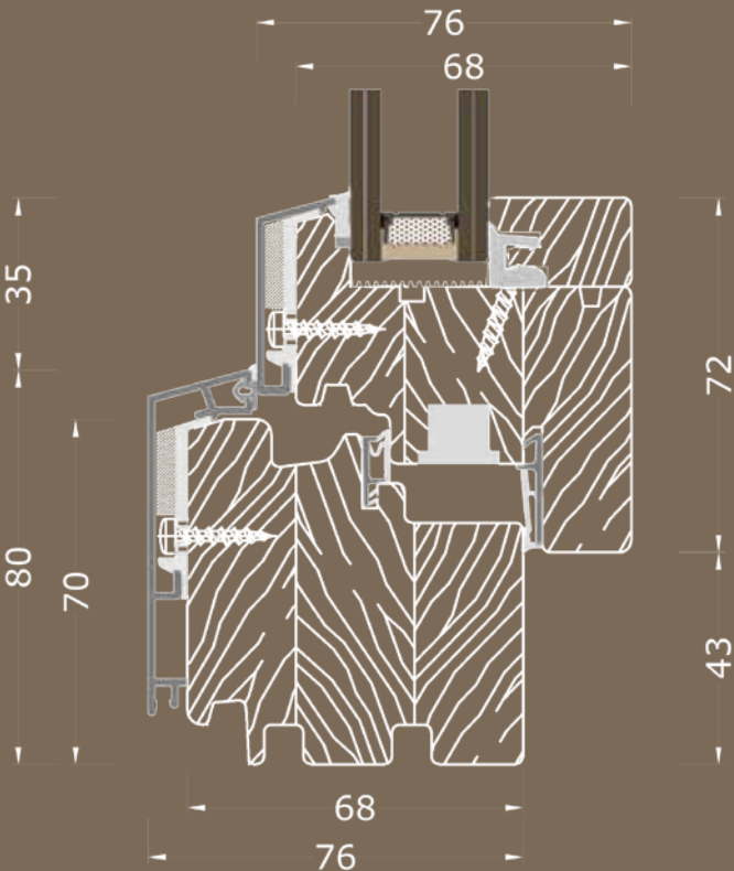
NODO INFERIORE
